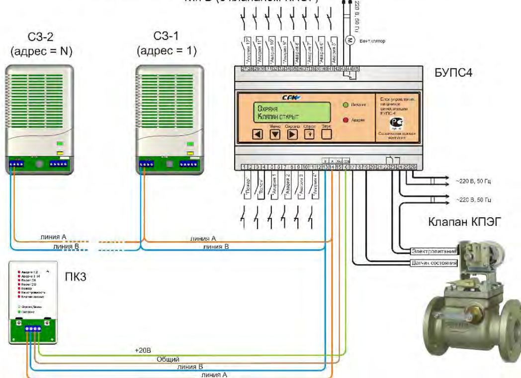
Система автономного контроля загазованности с диспетчеризацией тип Б (с клапаном КПЭГ)
